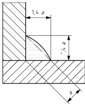
Εικόνα 1.3 Διαστάσεις εξωρραφών
