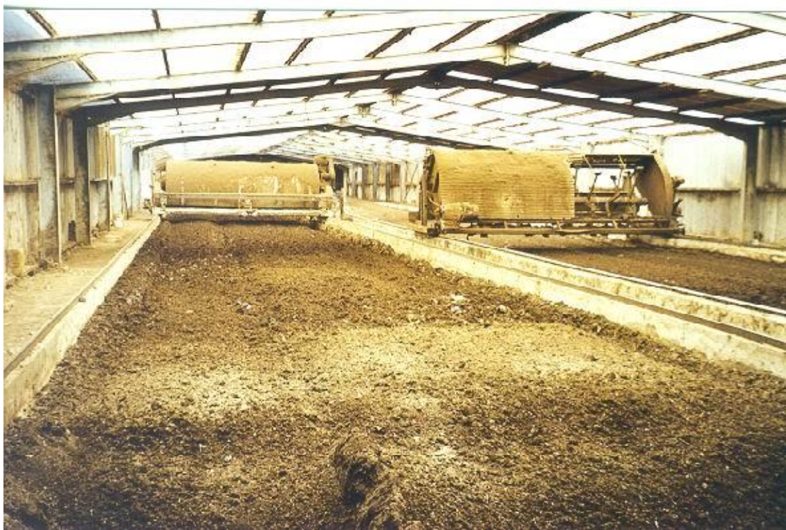
Σχήμα 5. Εικόνα μηχανικά αναστρεφόμενων κομποστοσωρών στερεών αποβλήτων πτηνοτροφείου αυγοπαραγωγής (πηγή: Εργαστήριο Γεωργικών Κατασκευών του ΓΠΑ).
